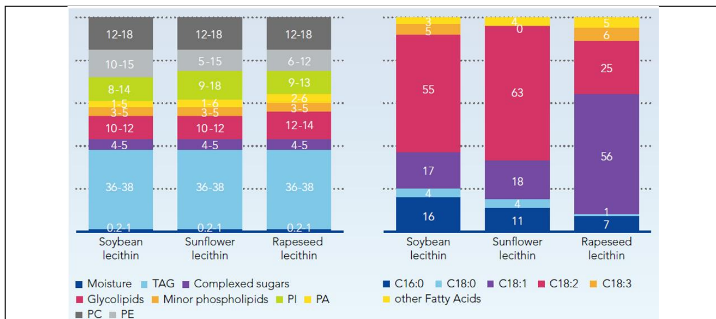
Figure 6 : La composition (à gauche) de quelques produits commercialisés sous le nom de « lécithine » (lécithine de soja, de tournesol, de colza). « Moisture » désigne l'eau présente ; les TAG sont les triglycérides ; les abréviations PI, PA, PC, PE signifient respectivement phosphatidylinositol, acide phosphatidique, phosphatidylcholine, phosphatidyléthanolamine. A droite, on a indiqué la proportion de divers résidus d'acides gras (fatty acids) : le nombre après la lettre C désigne la longueur de la chaîne, en nombre d'atomes de carbone ; le nombre après les deux points indique les insaturations, c'est-à-dire la présence éventuelle de doubles liaisons entre des atomes de carbone.
