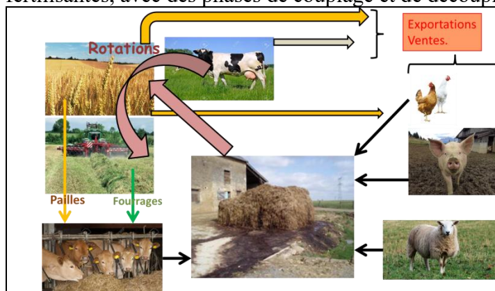
Figure 3 : l'exploitation de polyculture-élevage vue comme une unité métabolique bio-géochimique assurant les fonctions de couplage-découplage-recouplage des cycles C-N-P
