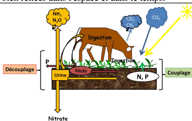
Figure 4 : limites à l'intensification des systèmes herbagers liées au seuil de chargement à partir duquel le découplage par l'animal excède les capacités de recouplage de la végétation.
